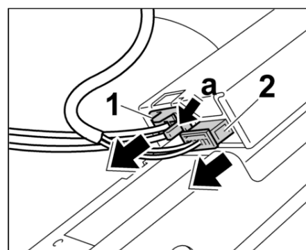
Scollegamento del conduttore ottico
