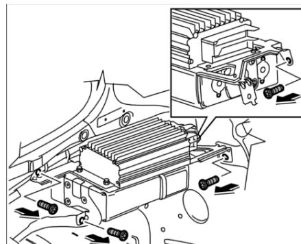
Rimozione delle viti di fissaggio del supporto
