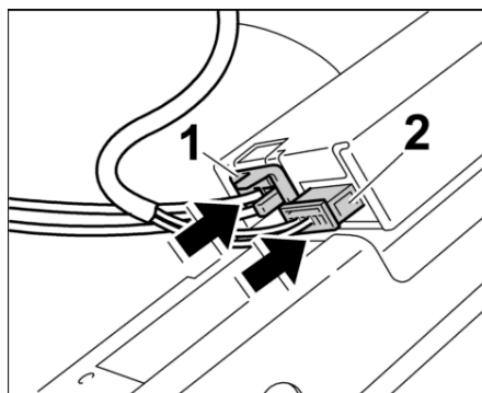
Inserimento conduttore ottico
