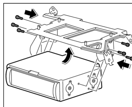
Viti di fissaggio cambia CD al supporto
