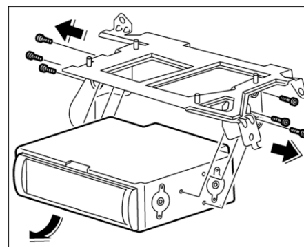
Rimozione delle viti di fissaggio del cambia CD
