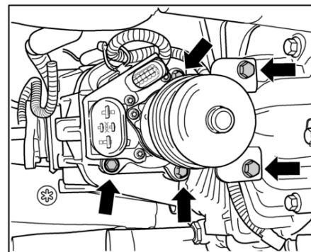
Avvitamento servomotorino
