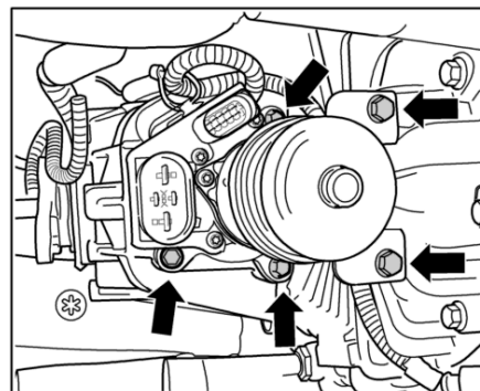
Avvitamento servomotorino
