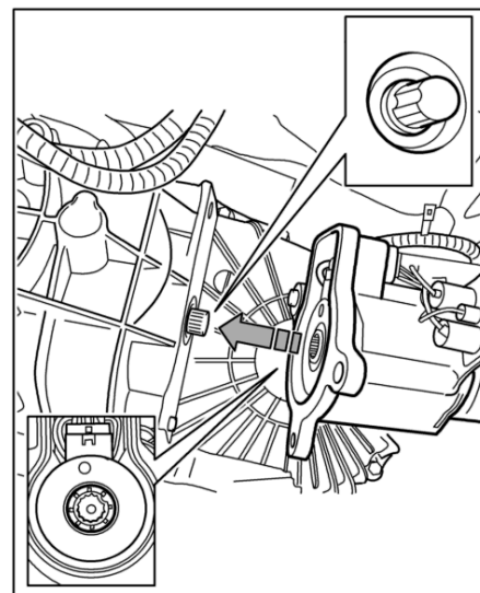
Posizionamento servomotorino
